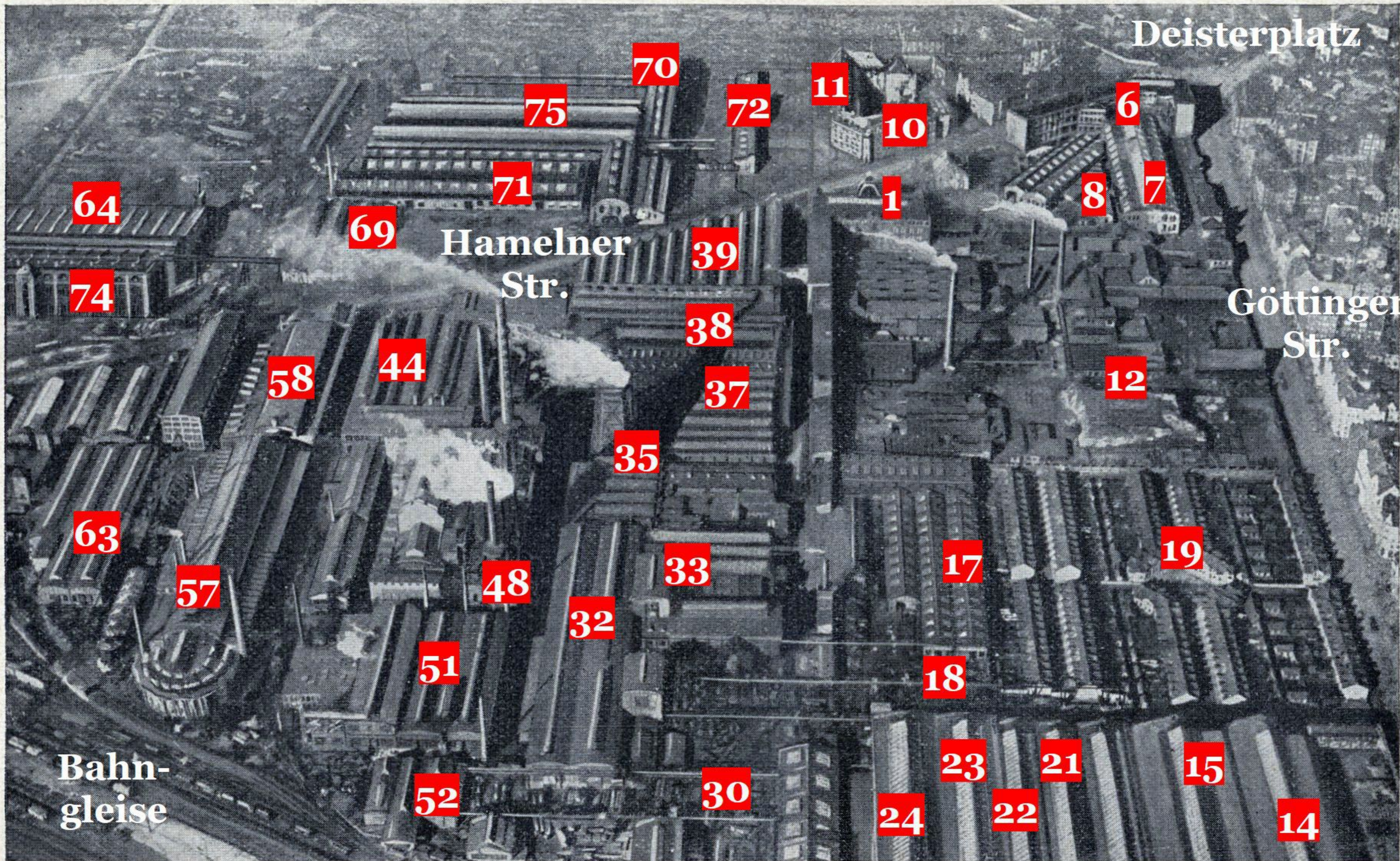
Abb. 10. Luftbild der Werksanlagen der Hanomag von der Bahnstrecke Hameln—Hannover, Bahnhof Vinden, aus gesehen. In der rechten oberen Ecke, im Winkel des Dreiecks am Deisterplatz liegen die Werkstätten des Schlepperbaus
