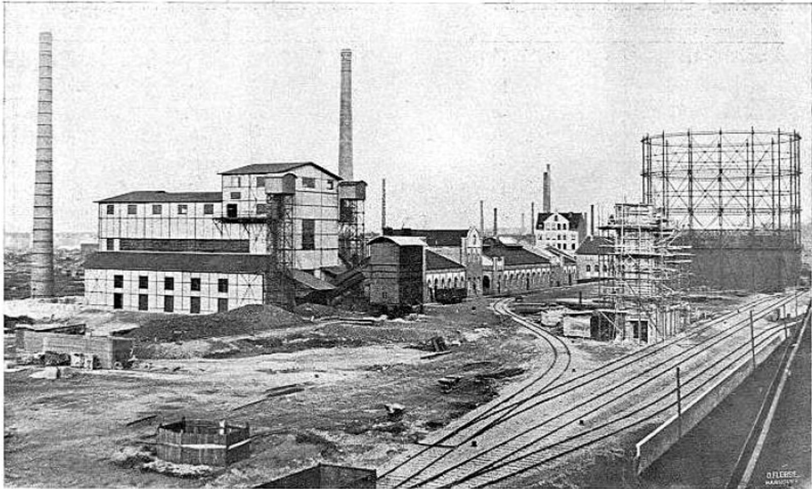
Gesamtansicht der Gasanstalt.
