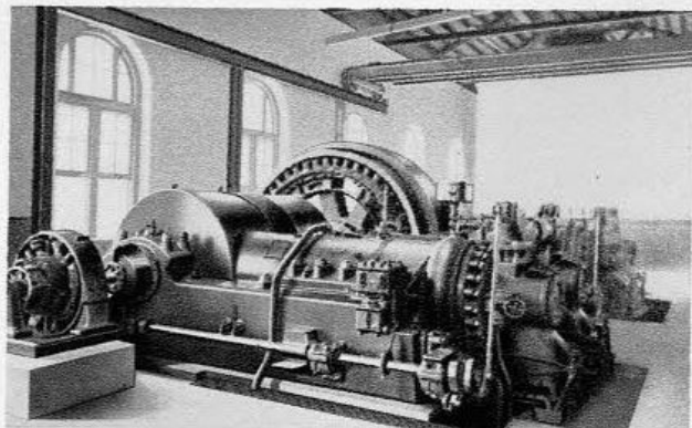
1000 PS Körtling-Dieselmotor ohne Kompressor liegender Bauart
