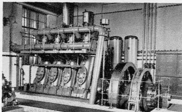
420 PS Körtling-Dieselmotor ohne Kompressor stehender Bauart
