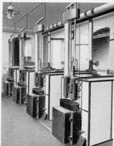
Körtling-Niederdruckdampfheizung
