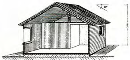
Decke = Dach 4 m oder 5 m breit Baureihe S 4 D=D oder S 5 D=D
